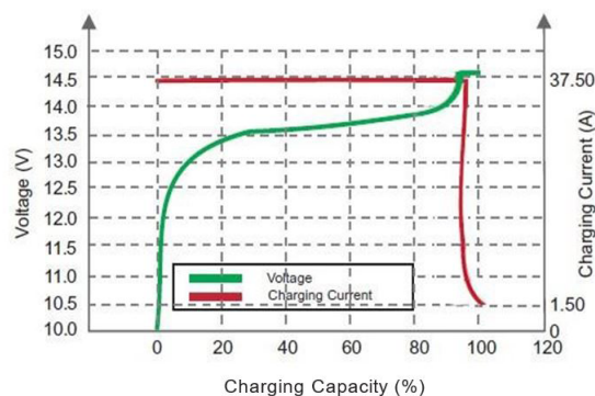
LADECHARAKTERISTIK (0.5C, 25 °C)
