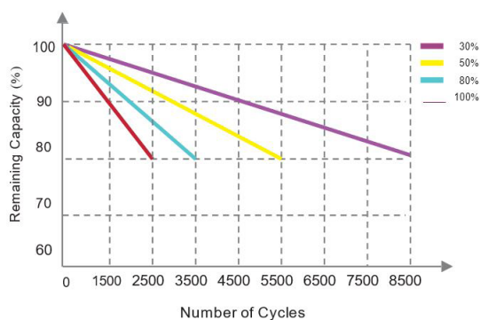
ZYKLENFESTIGKEIT IN RELATION ENTLADETIEFE
